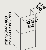
Optional chimney
