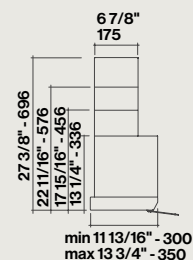
Optional chimney
